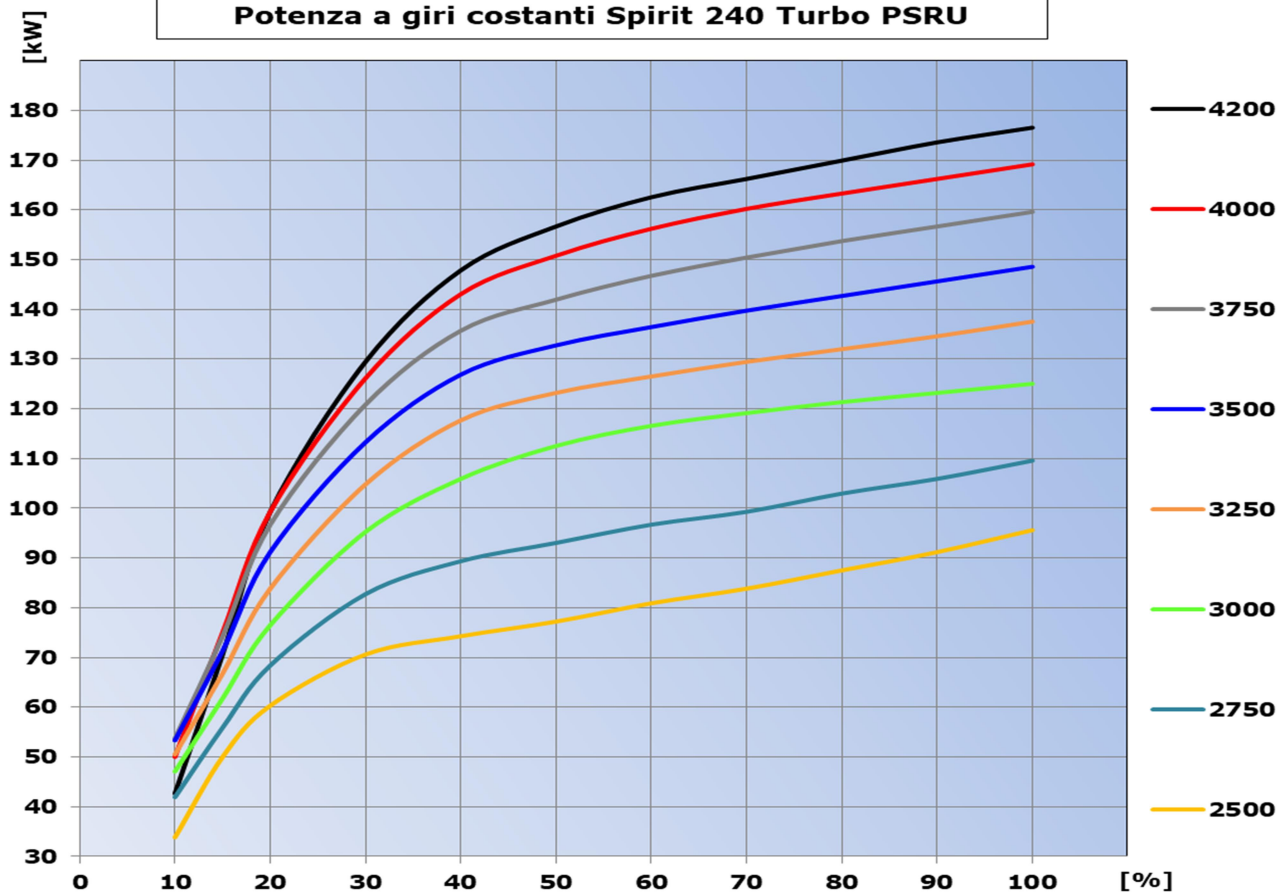
Potenza a giri costanti Spirit 240 Turbo PSRU
