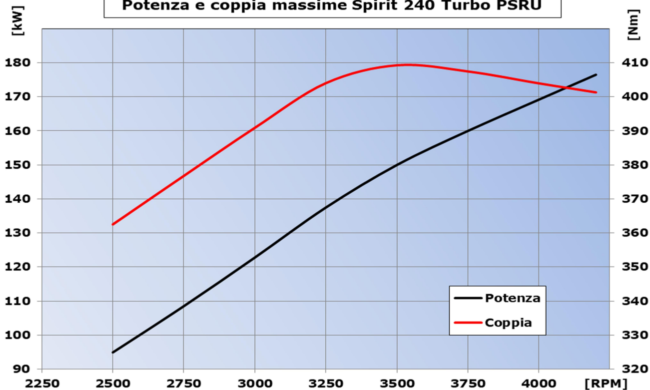
Potenza e coppia massime Spirit 240 Turbo PSRU
